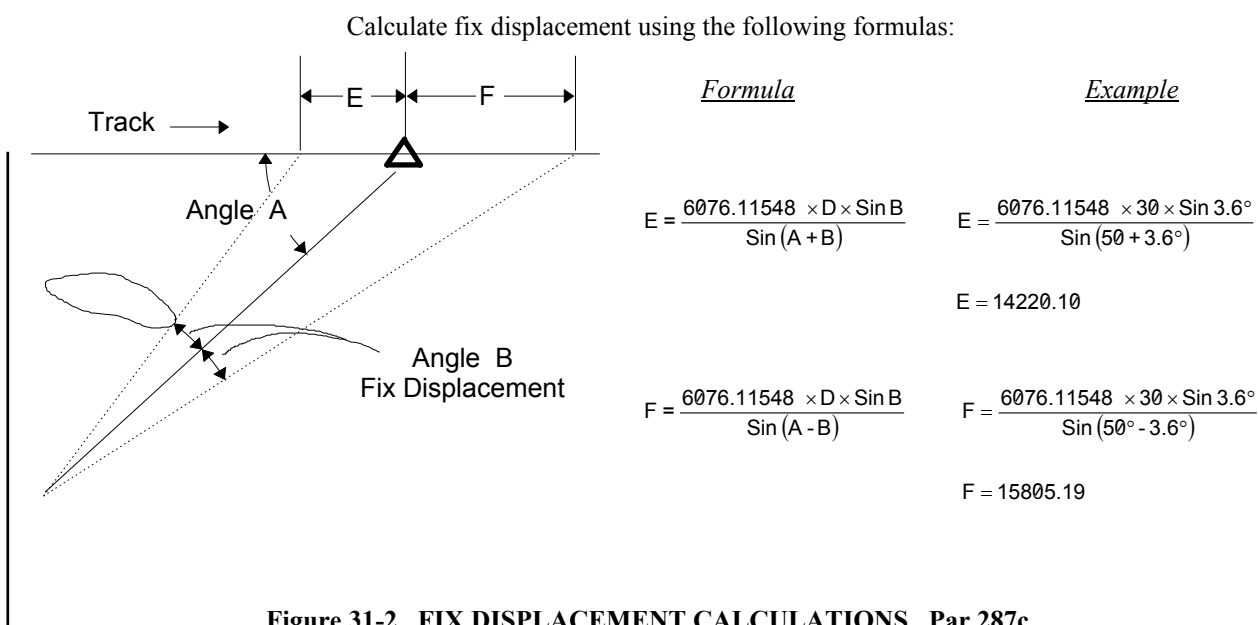
Figure 31-2. FIX DISPLACEMENT CALCULATIONS. Par 287c.
