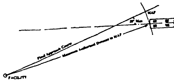
Figure 52. MAP. Off-Airport VOR with FAF. Par 514a(1).
