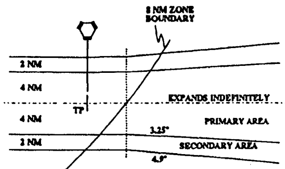
Figure 15-4. VOR/DME BASIC AREA. Par 1510a(1)
