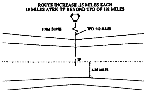
Figure 15-5. VOR/DME BASIC AREA. Par 1510a(1) and b(1).
