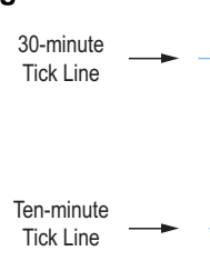
Figure 3.52 Latitude
