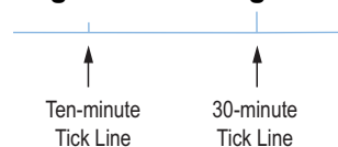
Figure 3.53 Longitude
