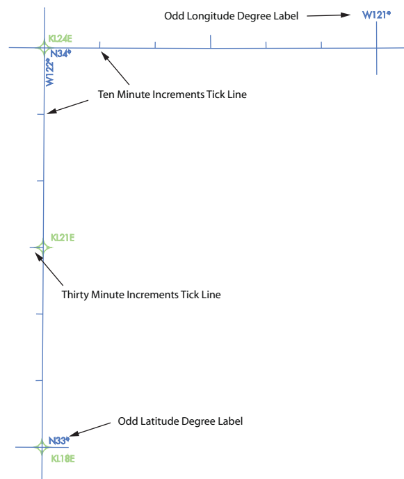
Figure 3.36 Latitude and Longitude Increments and Labels
