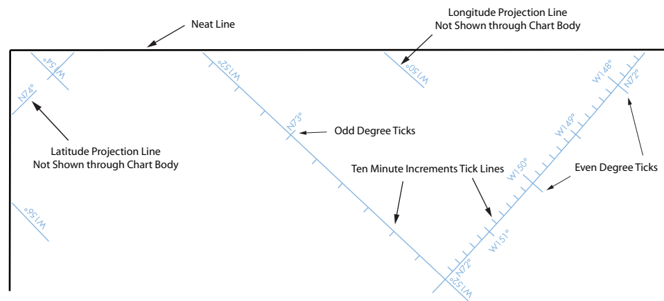
Figure 3.37 (AK) Latitude and Longitude Increments and Labels
