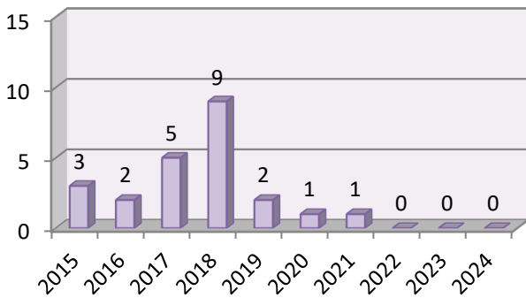
8. Improper Flare
