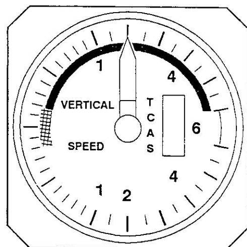
(d) Corrective REDUCE CLIMB.
