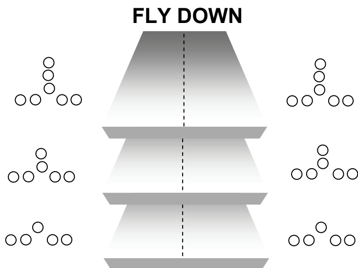
Figure 7-11. T-VASI.
