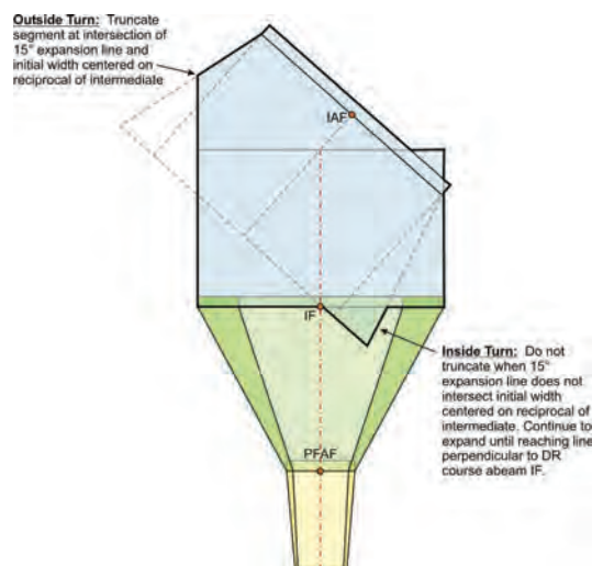
Figure 4-5. EXAMPLE DR SEGMENT. Par 233b.
