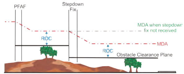
Figure 35. FINAL SEGMENT STEPDOWN FIX. Par 288c.
