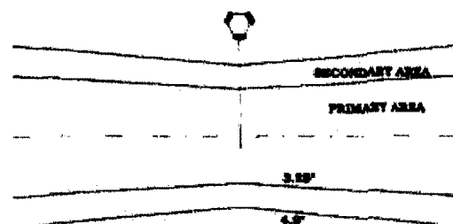
Figure 15-11. VOR/DME SECONDARY AREAS SPRAY 4.9°. Par 1512b(2)(a).
