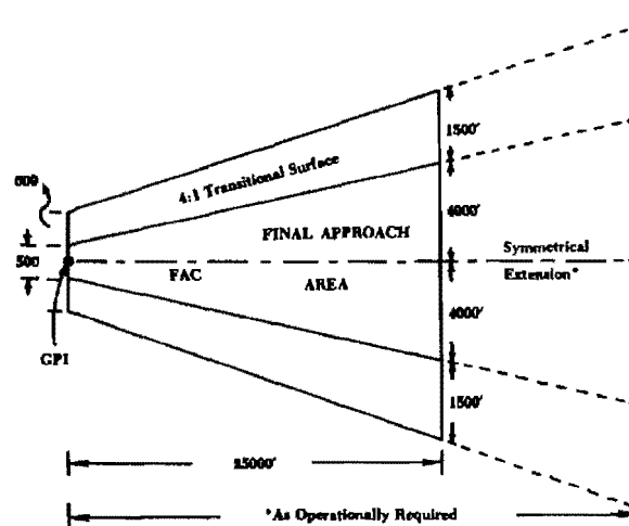
Figure 110. PAR FINAL APPROACH AREA. Par 1159 and 1160
