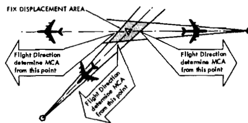
Figure 17-21. DETERMINATION OF MCA Par 1730.
