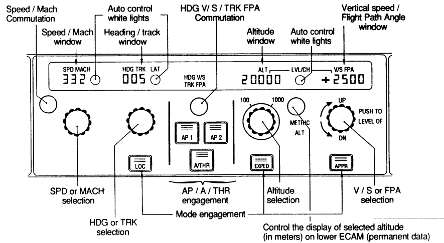
Airbus A320
