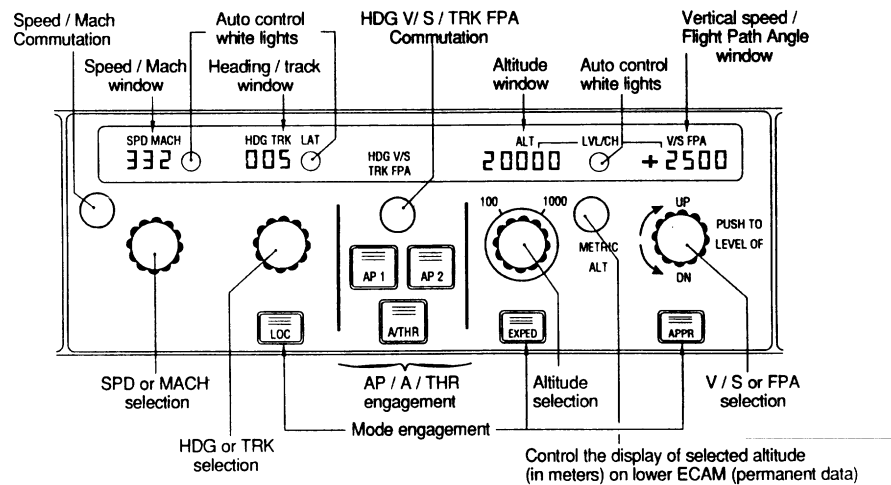
Airbus A320
