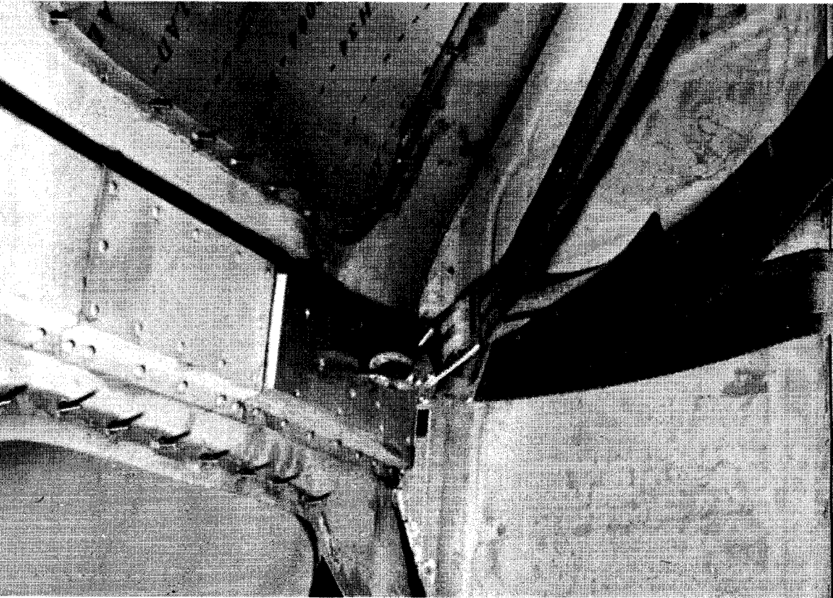
FIGURE 7. Ercoupe.
